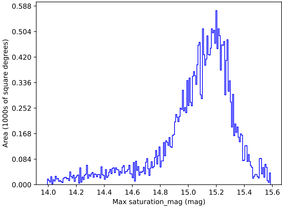
weather_cloudso30v3.4_10yrs All sky z band: Max saturation_mag
