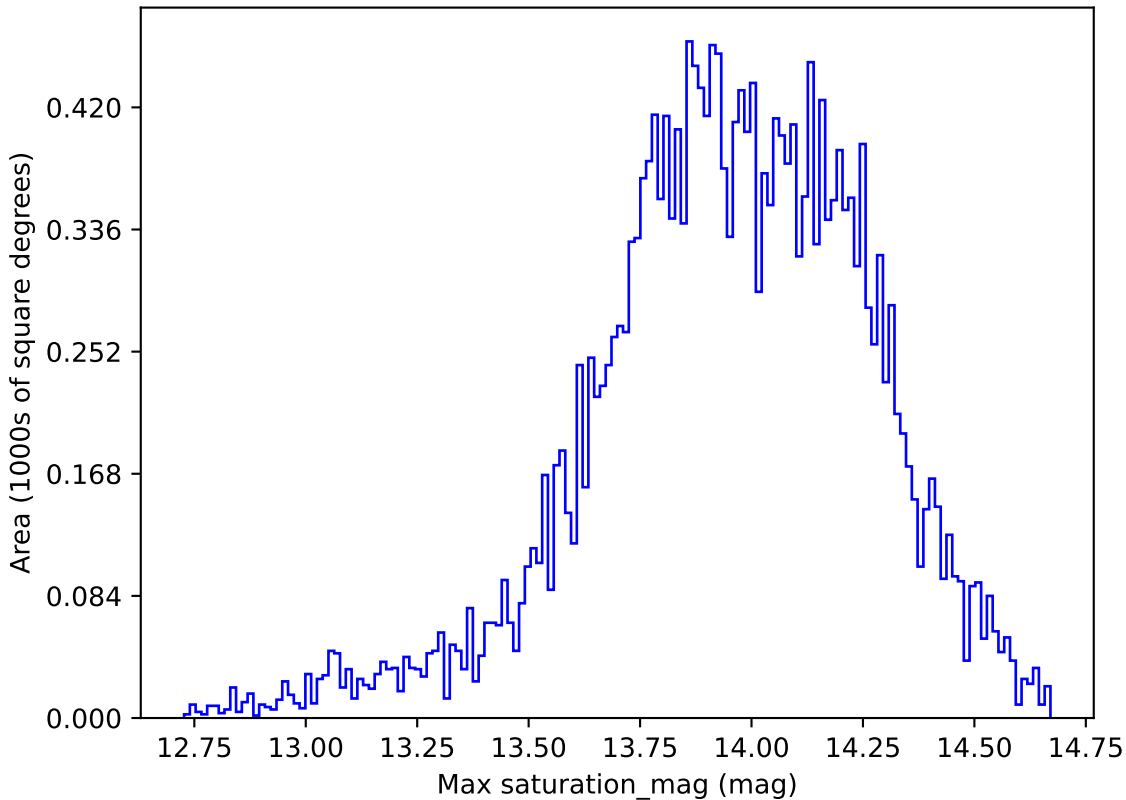
weather_cloudso30v3.4_10yrs All sky u band: Max saturation_mag
