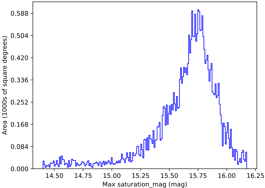
weather_cloudso30v3.4_10yrs All sky r band: Max saturation_mag
