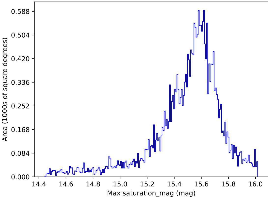
weather_cloudso30v3.4_10yrs All sky i band: Max saturation_mag
