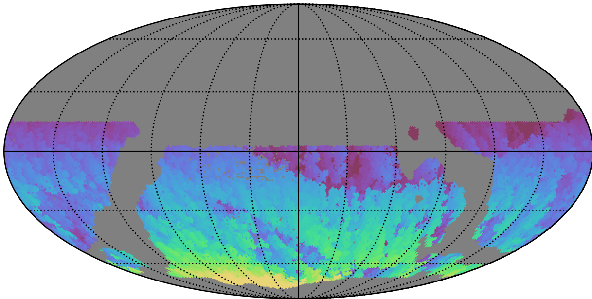
weather_cloudso30v3.4_10yrs WFD i band: Max HA
