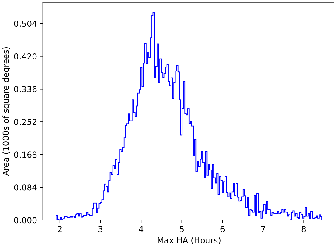
weather_cloudso30v3.4_10yrs All sky y band: Max HA
