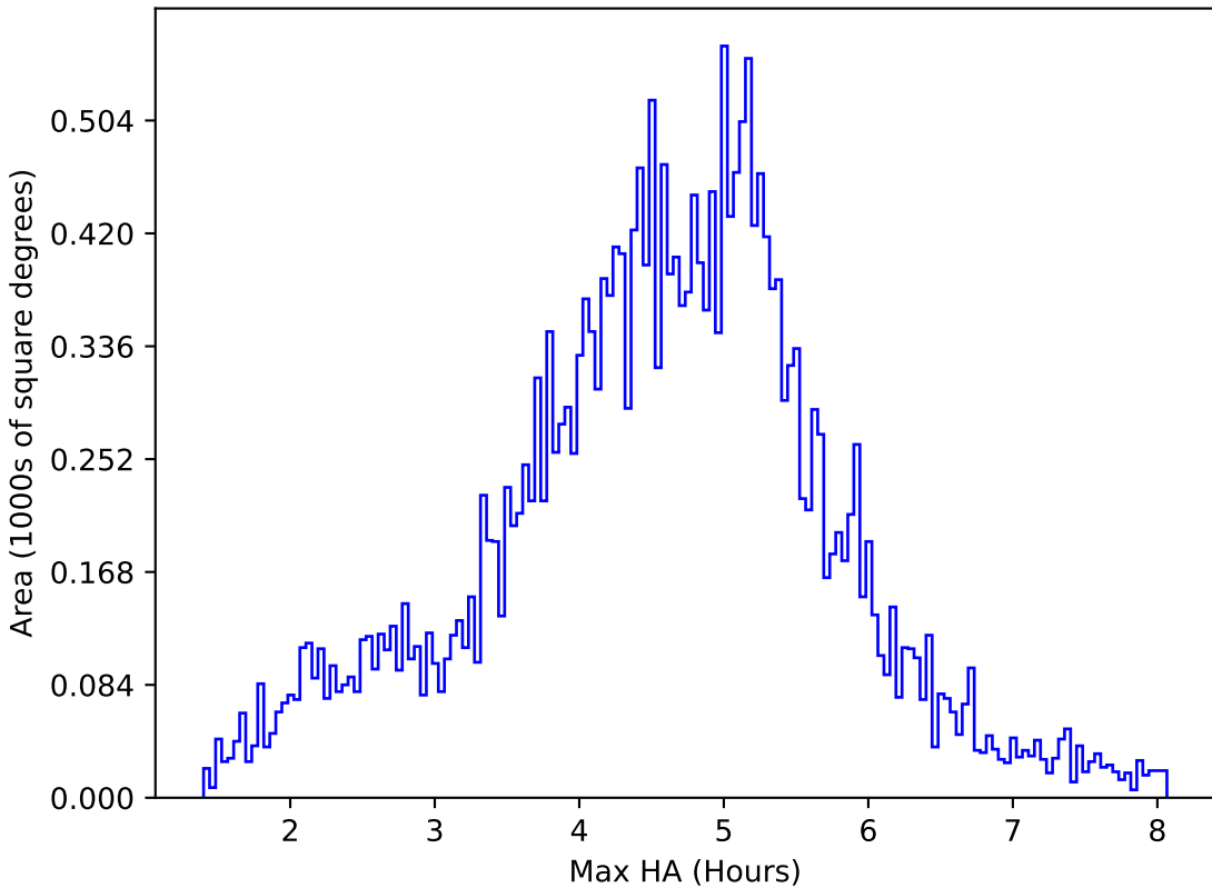
weather_cloudso30v3.4_10yrs All sky i band: Max HA
