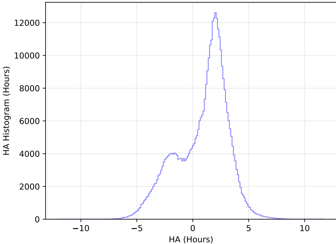
weather_cloudso30v3.4_10yrs WFD y band: HA Histogram
