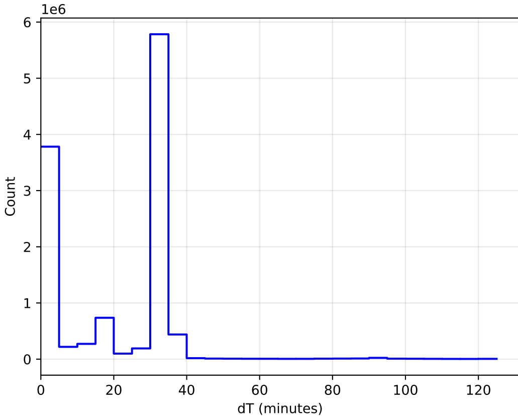
weather_cloudso30v3.4_10yrs WFD: DeltaT Histogram
