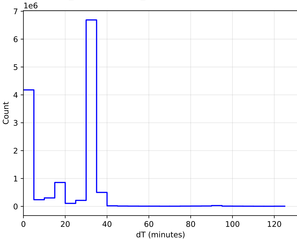
weather_cloudso30v3.4_10yrs All sky: DeltaT Histogram
