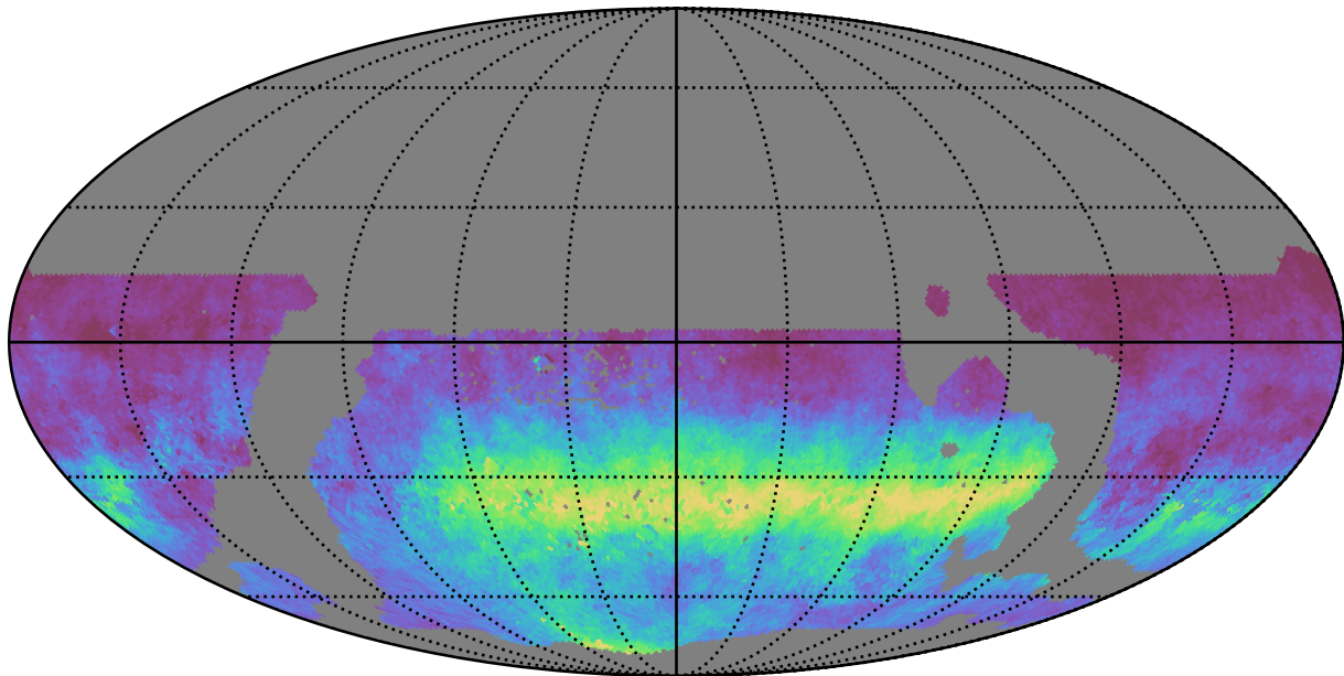
weather_cloudso30v3.4_10yrs WFD i band: AngleRms rotSkyPos
