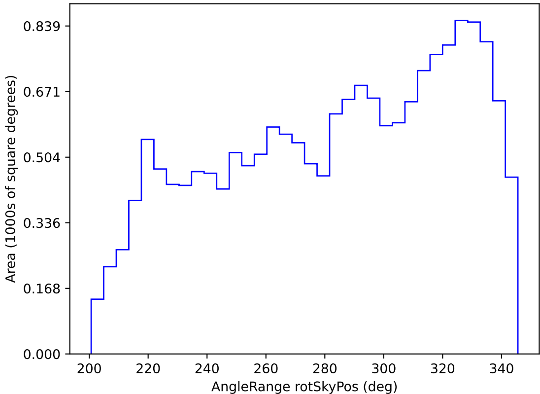
weather_cloudso30v3.4_10yrs WFD r band: AngleRange rotSkyPos
