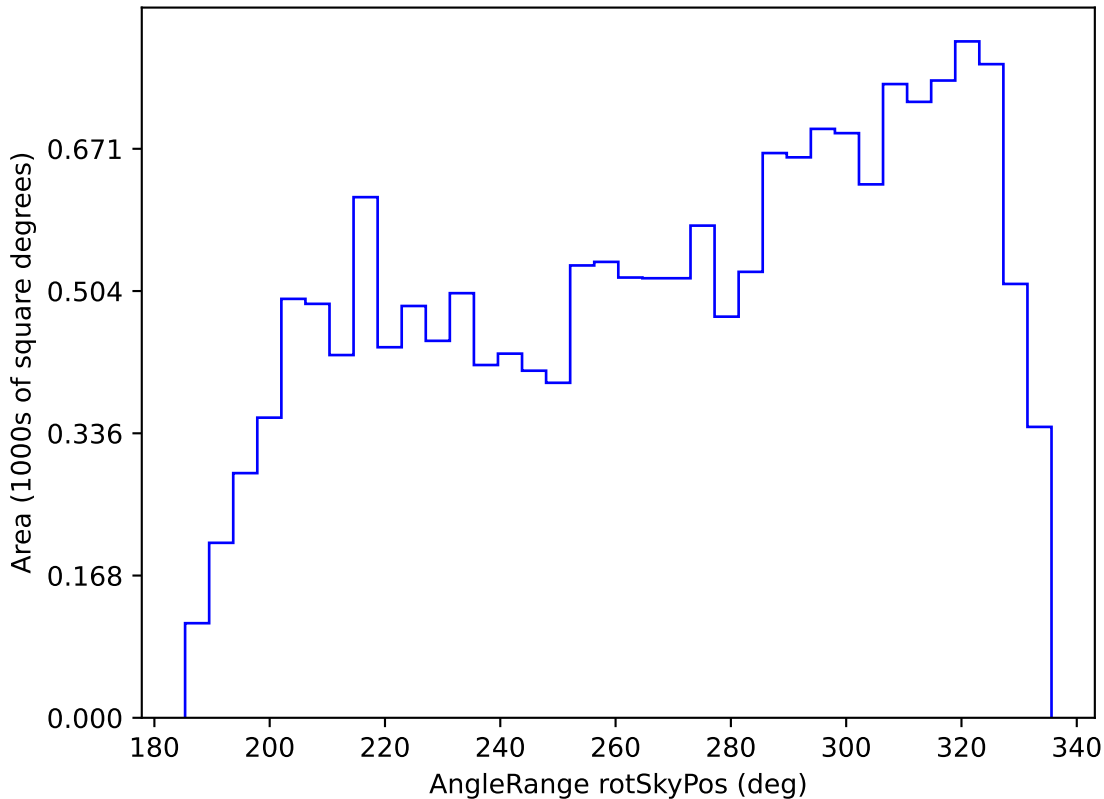
weather_cloudso30v3.4_10yrs WFD g band: AngleRange rotSkyPos
