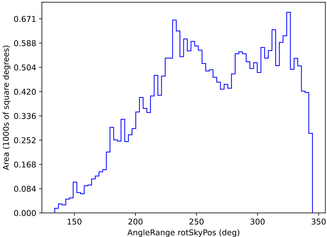
weather_cloudso30v3.4_10yrs All sky z band: AngleRange rotSkyPos
