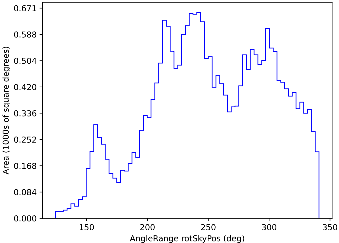
weather_cloudso30v3.4_10yrs All sky y band: AngleRange rotSkyPos
