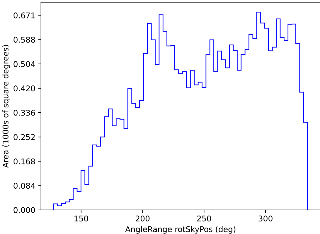
weather_cloudso30v3.4_10yrs All sky g band: AngleRange rotSkyPos
