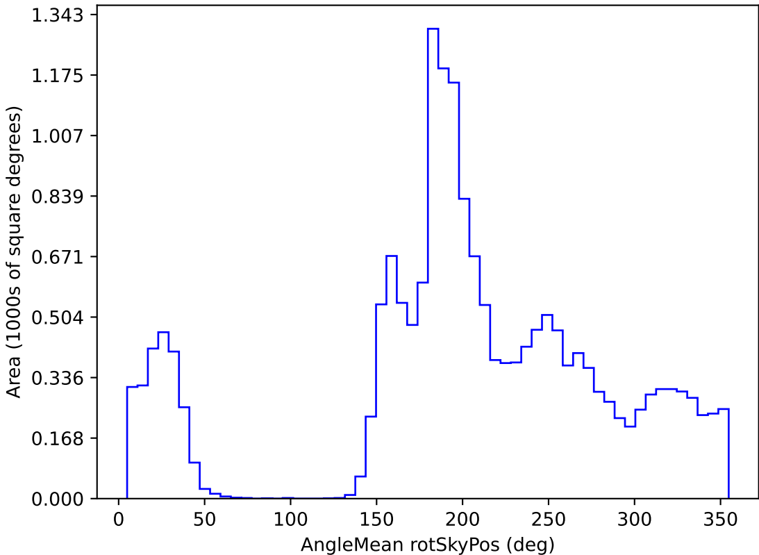
weather_cloudso30v3.4_10yrs WFD y band: AngleMean rotSkyPos
