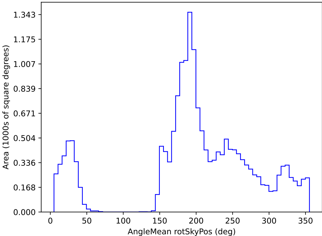
weather_cloudso30v3.4_10yrs WFD i band: AngleMean rotSkyPos
