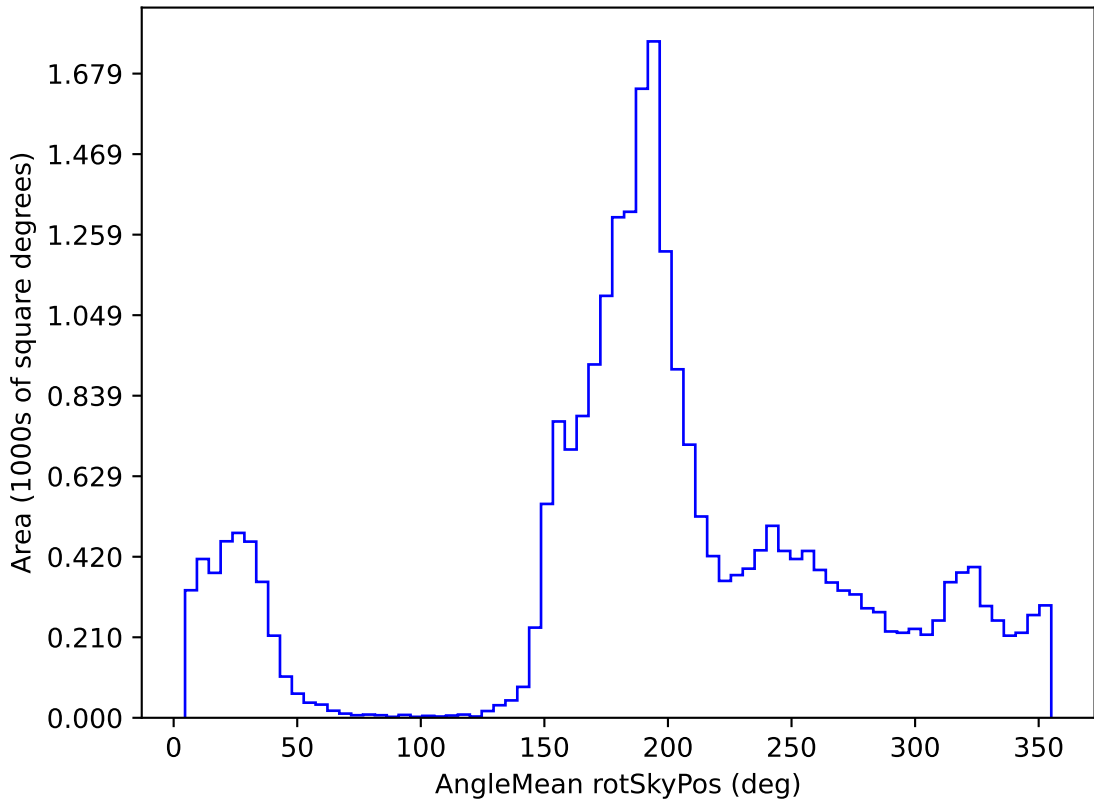
weather_cloudso30v3.4_10yrs All sky i band: AngleMean rotSkyPos
