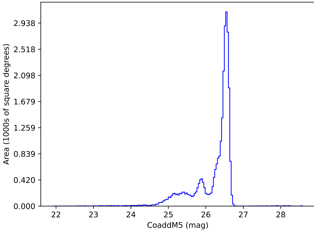
weather_cloudso30v3.4_10yrs i: CoaddM5
