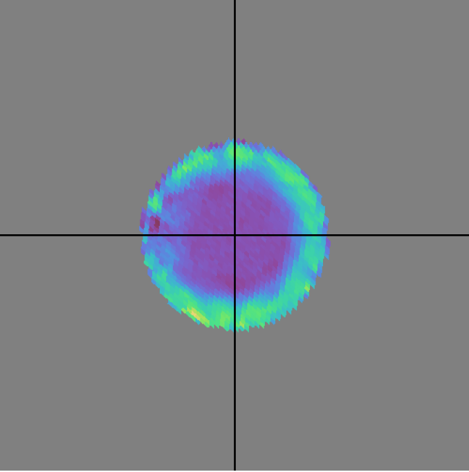
0.12 0.16 0.20 0.24 0.28 0.32 0.36 0.40 0.48 Kuiper statistic (0 is uniform, 1 is delta function),rotSkyPos,DD:ELAISS1,gri (deg)
