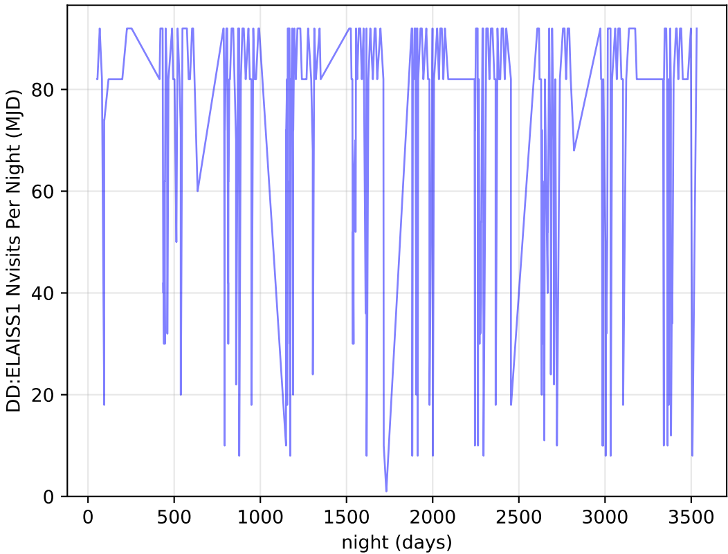
weather_cloudso30v3.4_10yrs all bands: DD:ELAISS1 Nvisits Per Night
