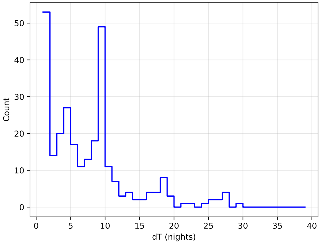
weather_cloudso30v3.4_10yrs all bands: DD:ELAISS1 Delta Nights Histogram
