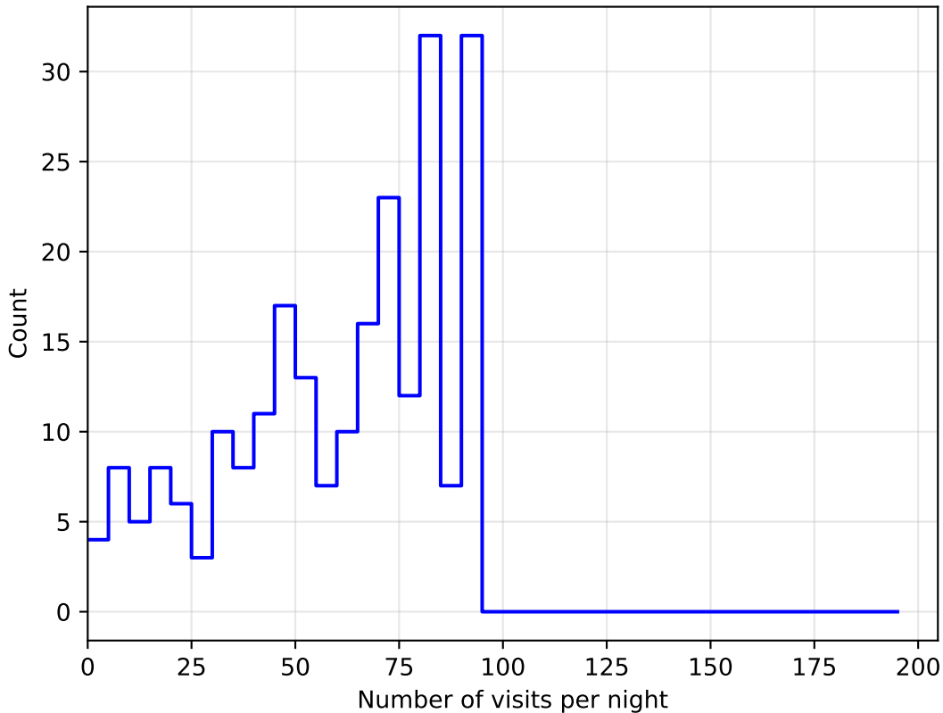
weather_cloudso30v3.4_10yrs all bands: DD:EDFS NVisitsPerNight
