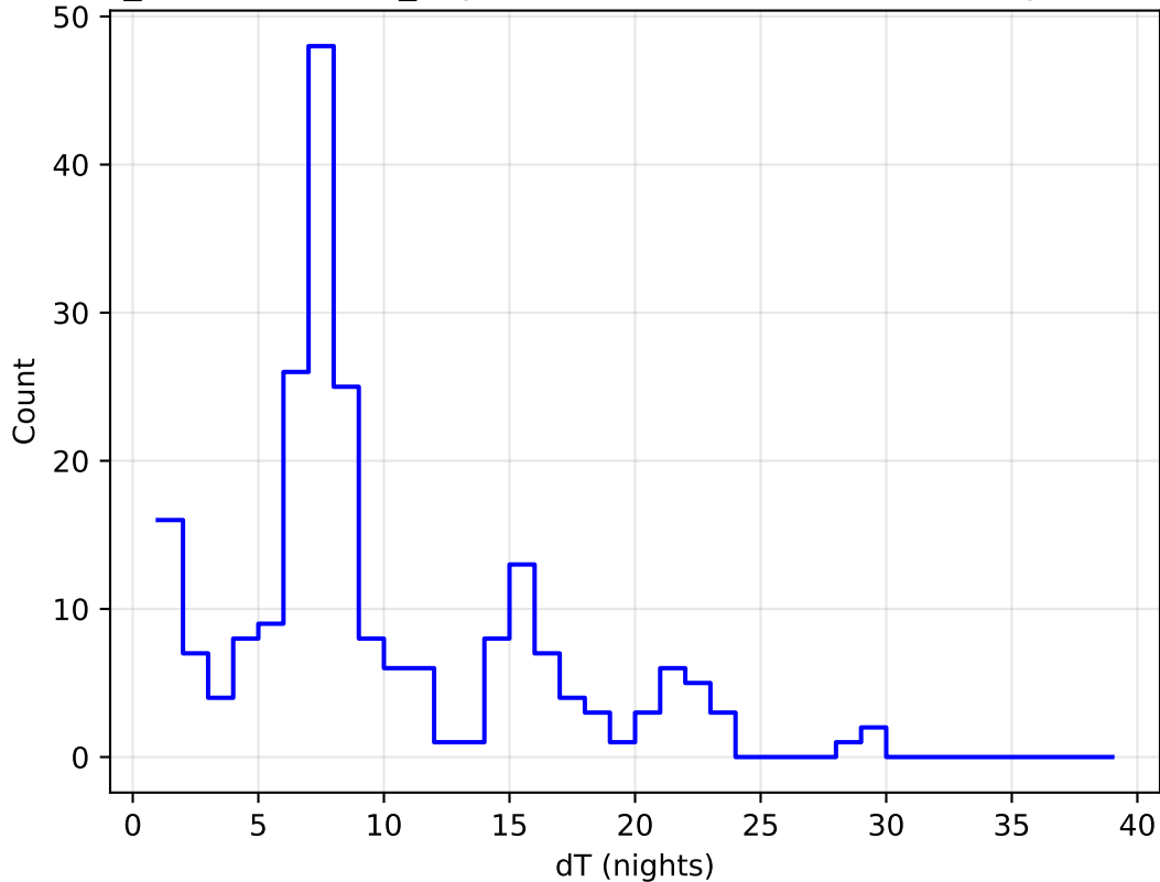
weather_cloudso30v3.4_10yrs all bands: DD:EDFS Delta Nights Histogram
