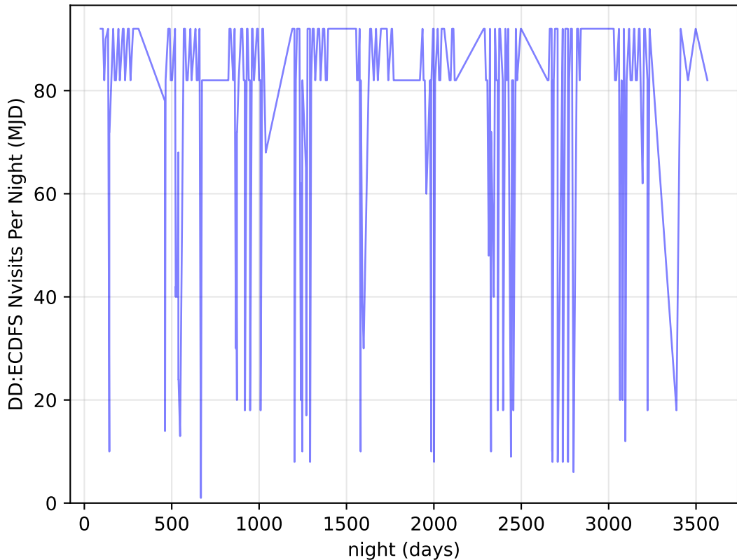
weather_cloudso30v3.4_10yrs all bands: DD:ECDFS Nvisits Per Night
