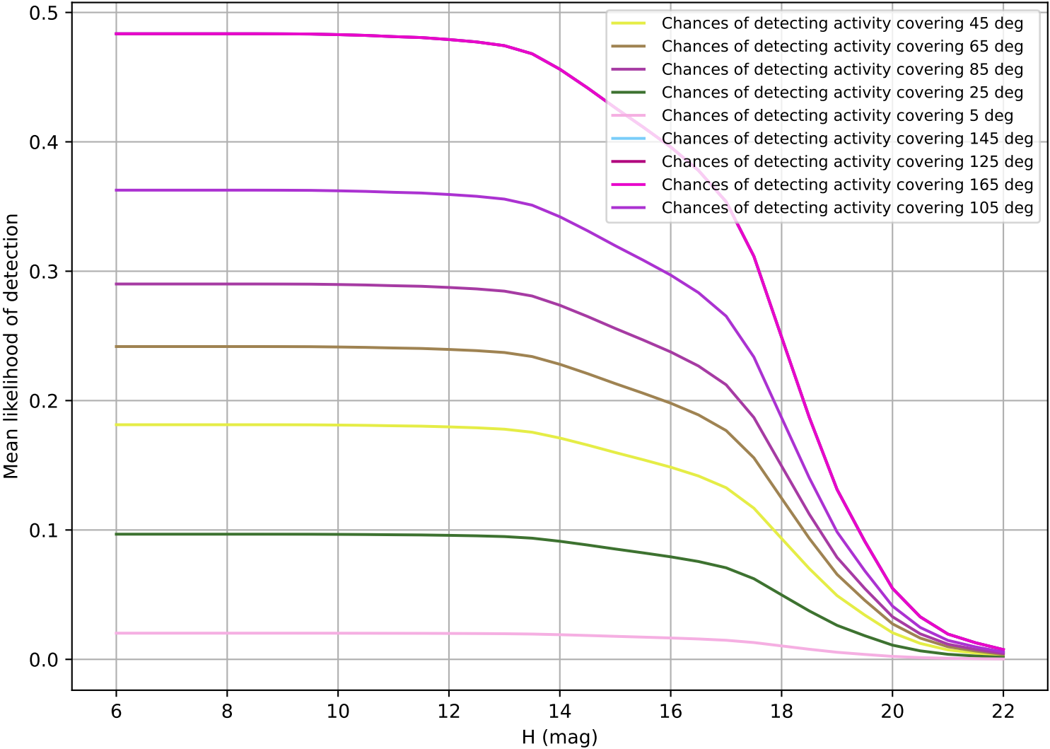
weather_cloudso2v3.4_10yrs OCC_r5
