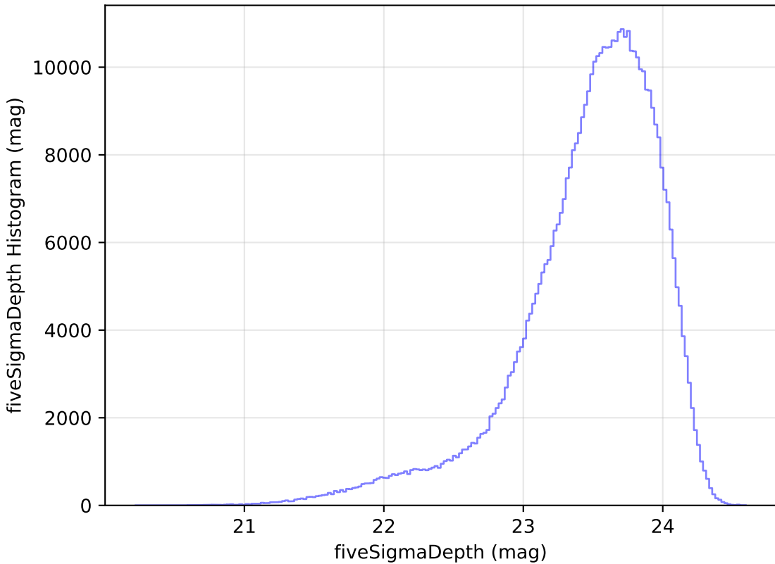
weather_cloudso2v3.4_10yrs i: fiveSigmaDepth Histogram
