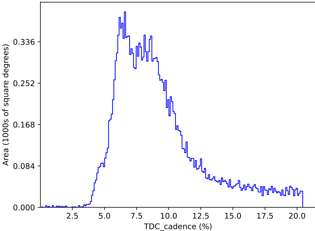
weather_cloudso2v3.4_10yrs : TDC_cadence
