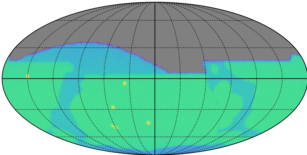
weather_cloudso2v3.4_10yrs i: SurfaceBrightLimit
