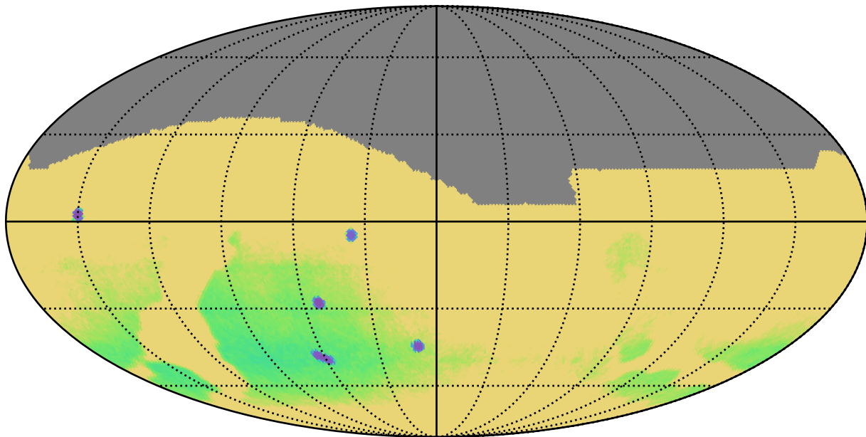
weather_cloudso2v3.4_10yrs : Parallax Uncert @ 22.4
