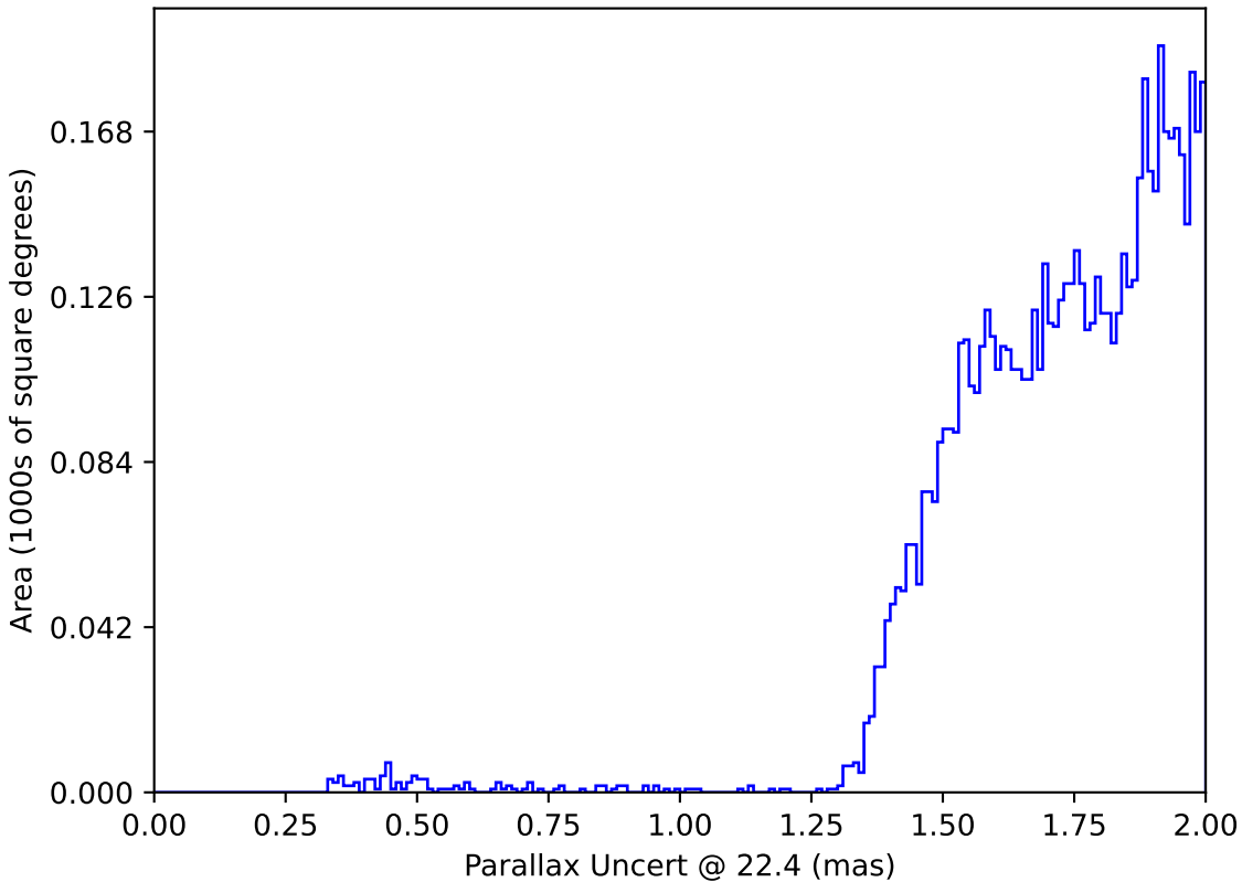
weather_cloudso2v3.4_10yrs : Parallax Uncert @ 22.4
