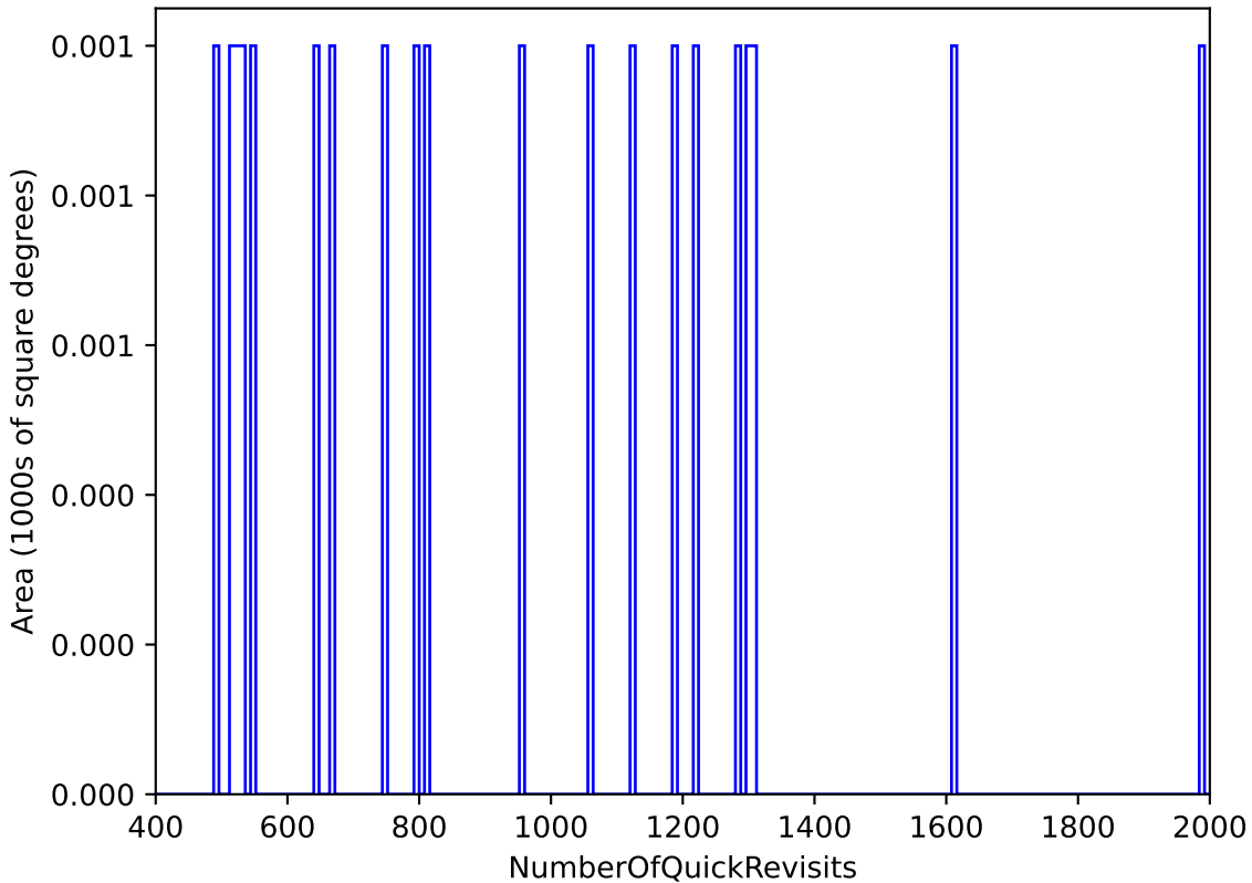
weather_cloudso2v3.4_10yrs : NumberOfQuickRevisits
