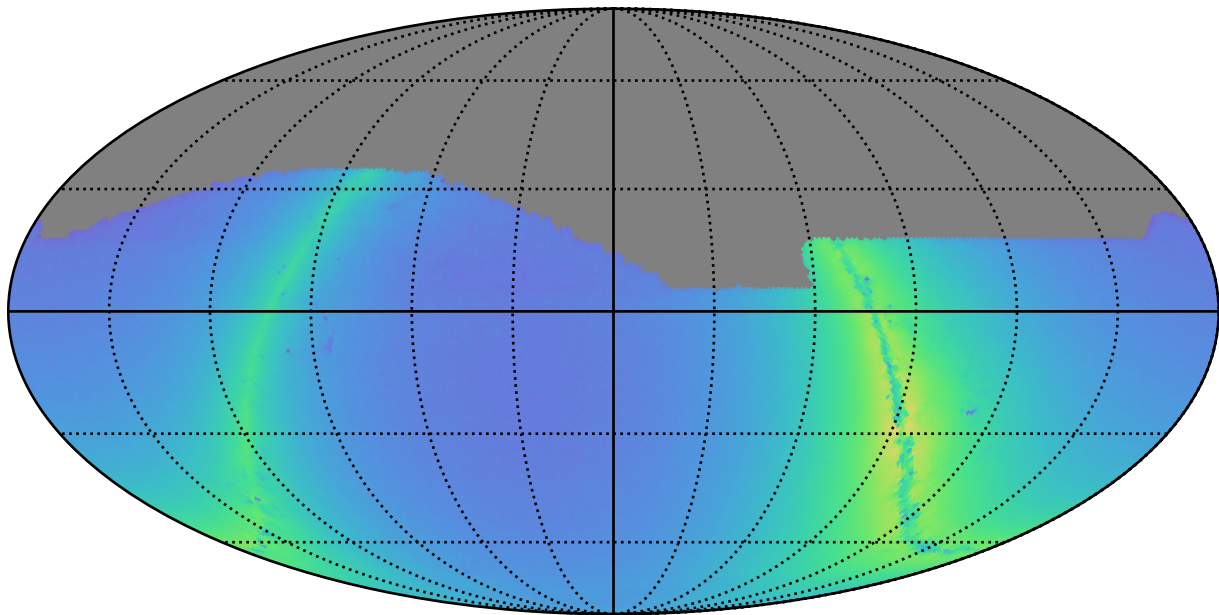
weather_cloudso2v3.4_10yrs z: Nstars_no_crowding
