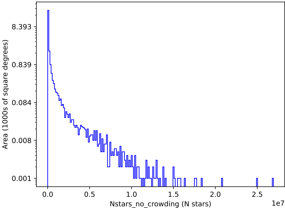
weather_cloudso2v3.4_10yrs z: Nstars_no_crowding
