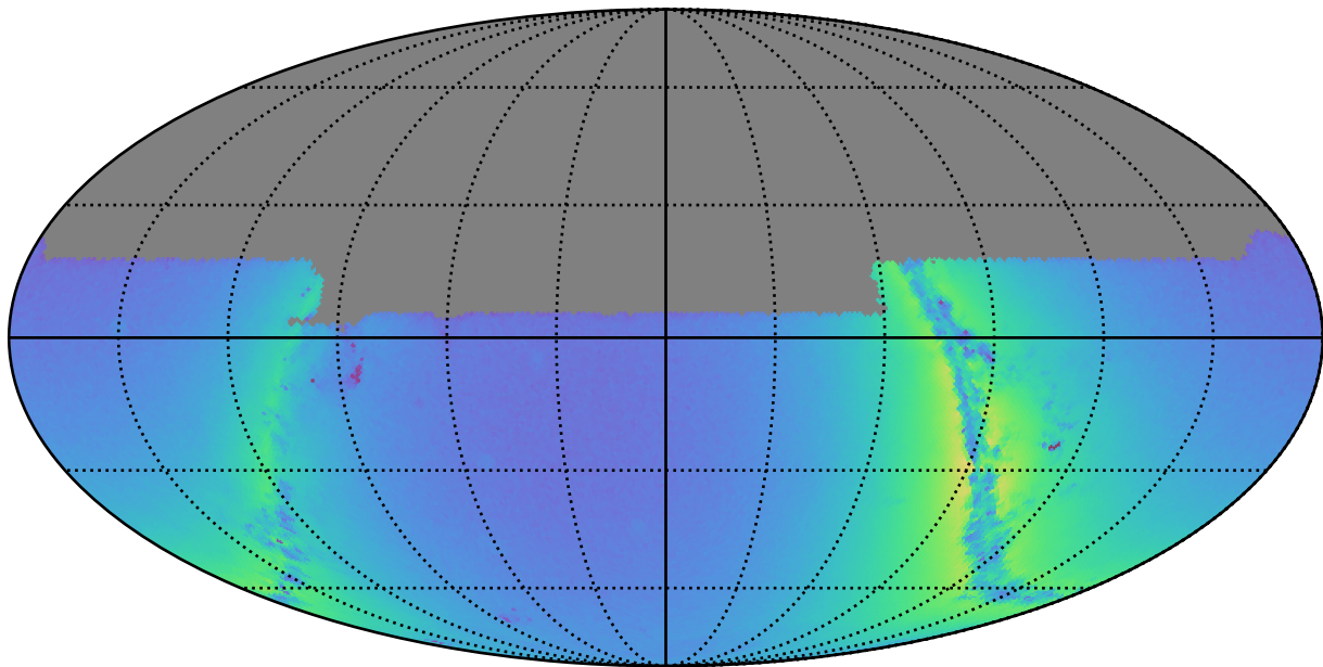
weather_cloudso2v3.4_10yrs u: Nstars_no_crowding
