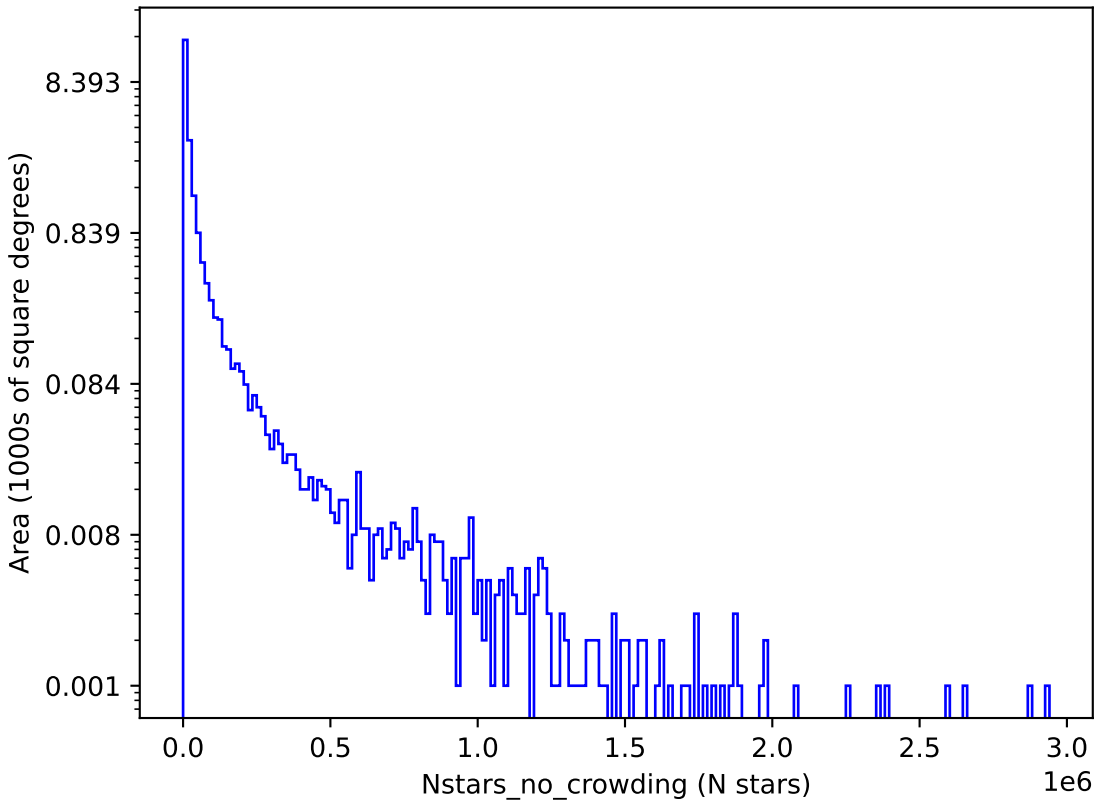
weather_cloudso2v3.4_10yrs u: Nstars_no_crowding
