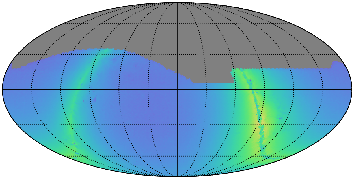
weather_cloudso2v3.4_10yrs r: Nstars_no_crowding
