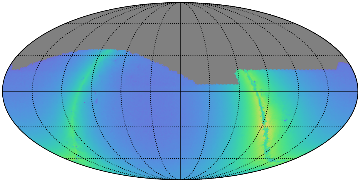
weather_cloudso2v3.4_10yrs i: Nstars_no_crowding
