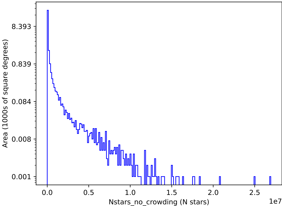
weather_cloudso2v3.4_10yrs i: Nstars_no_crowding
