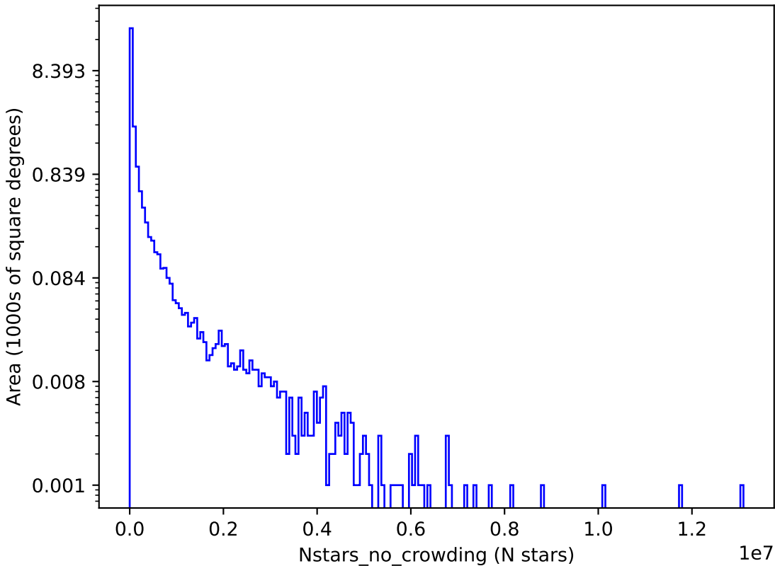
weather_cloudso2v3.4_10yrs g: Nstars_no_crowding
