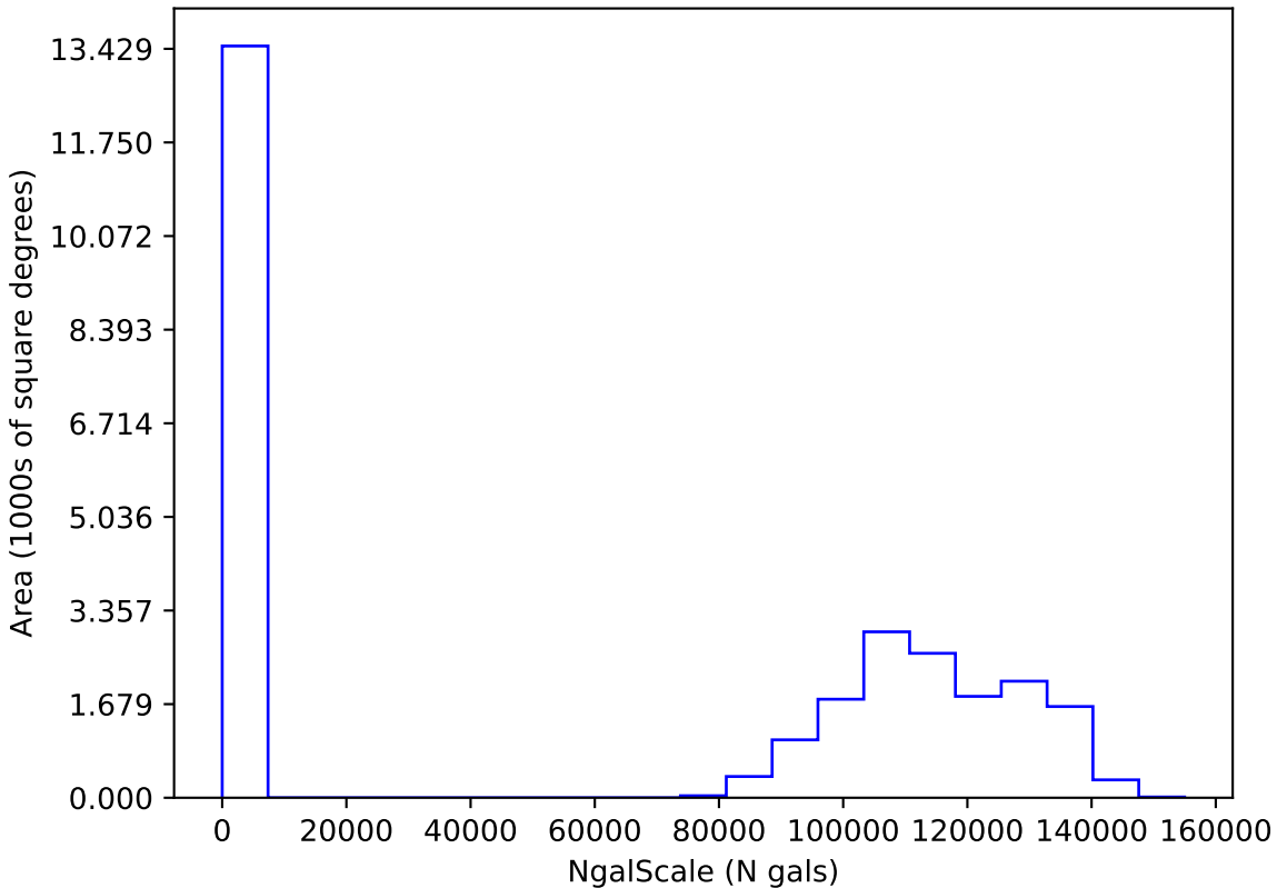
weather_cloudso2v3.4_10yrs i: NgalScale
