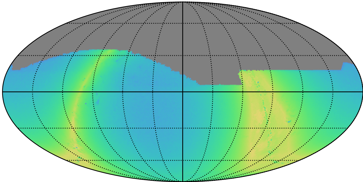
weather_cloudso2v3.4_10yrs i: N stars to Precision 0.20
