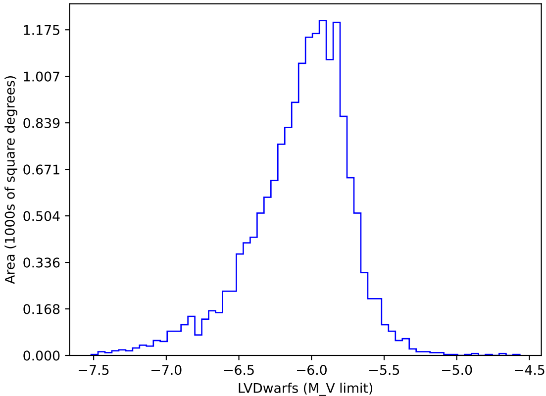
weather_cloudso2v3.4_10yrs gi: LVDwarfs
