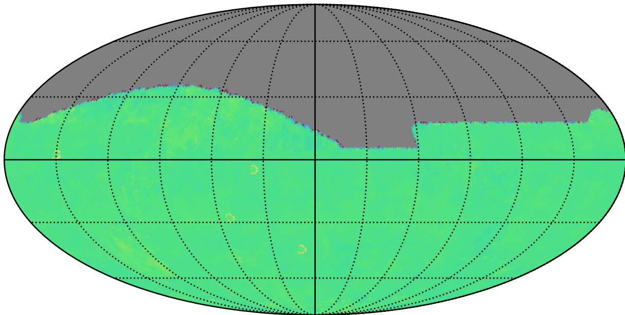
weather_cloudso2v3.4_10yrs z: Kuiper rotTelPos
