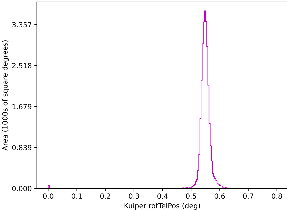
weather_cloudso2v3.4_10yrs z: Kuiper rotTelPos
