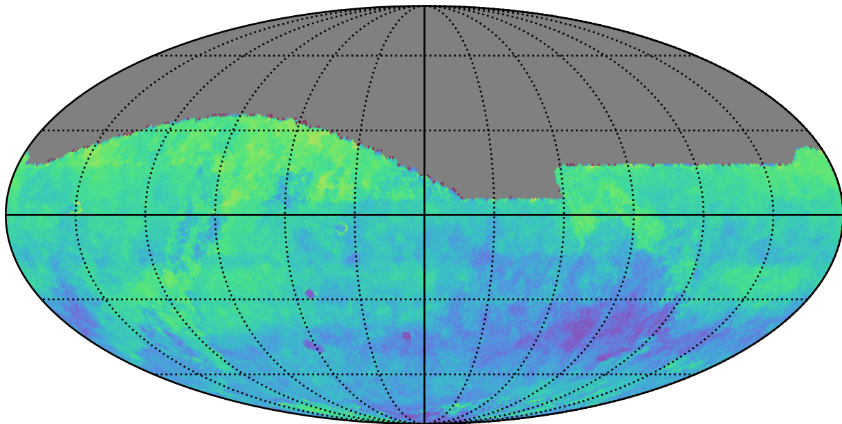
weather_cloudso2v3.4_10yrs z: Kuiper rotSkyPos
