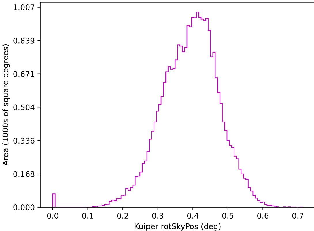
weather_cloudso2v3.4_10yrs z: Kuiper rotSkyPos
