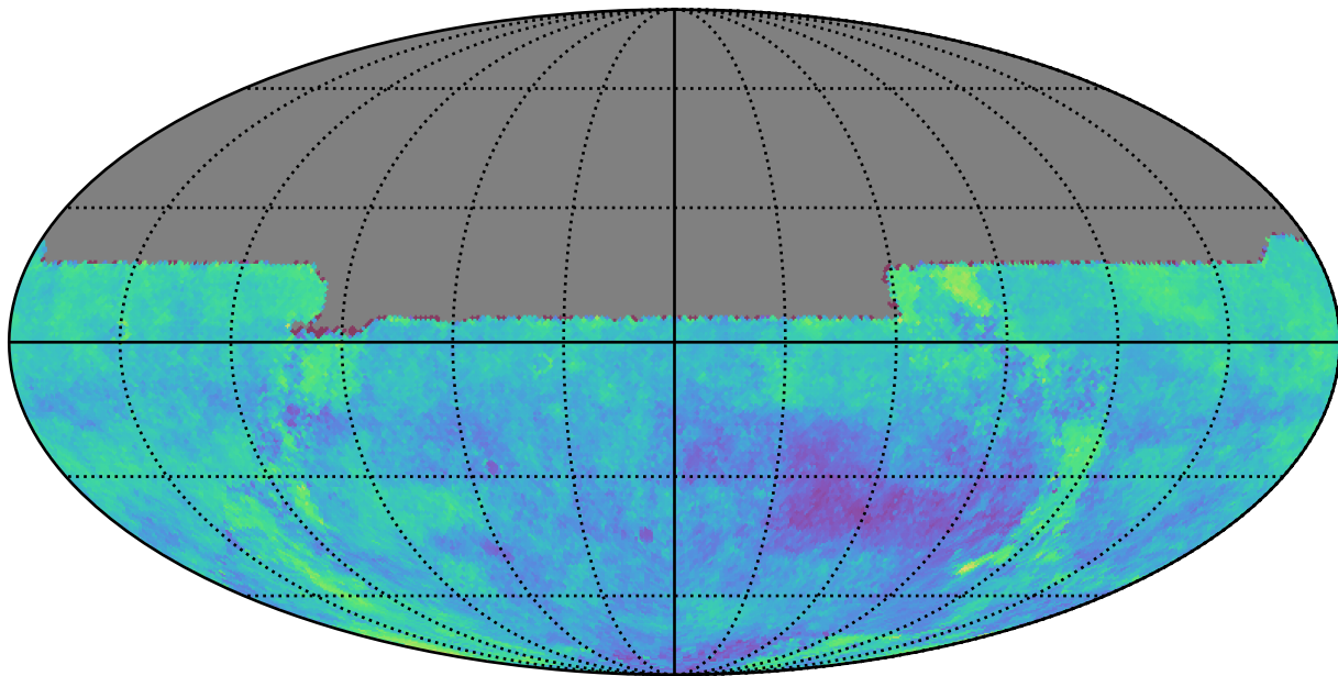
weather_cloudso2v3.4_10yrs u: Kuiper rotSkyPos
