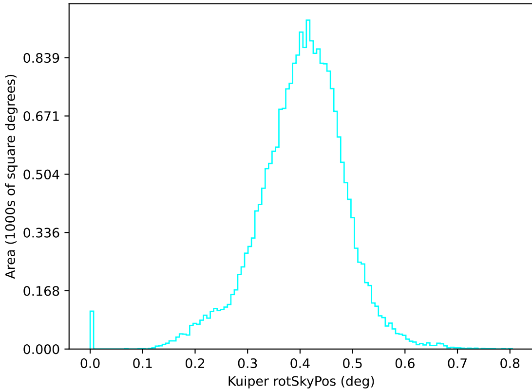
weather_cloudso2v3.4_10yrs u: Kuiper rotSkyPos
